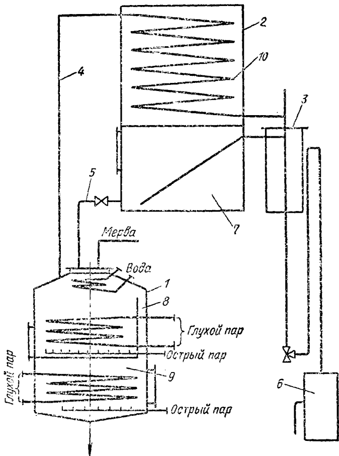
Рис. 38. Схема устройства воскоэкстракционного аппарата АВ-171
