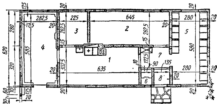
Рис. 56. План пчеловодной мастерской (размеры, мм)
