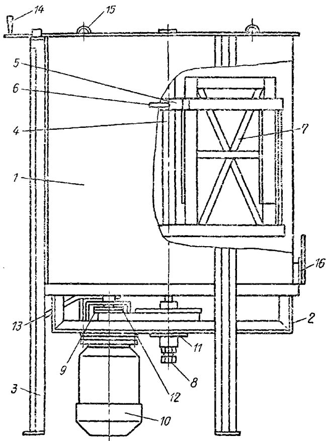
Рис. 32. Схема устройства медогонки электрифицированной М4.32.РЭ
