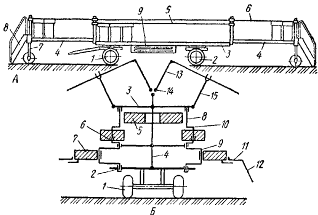
Рис. 54. Передвижные пасечные установки:
