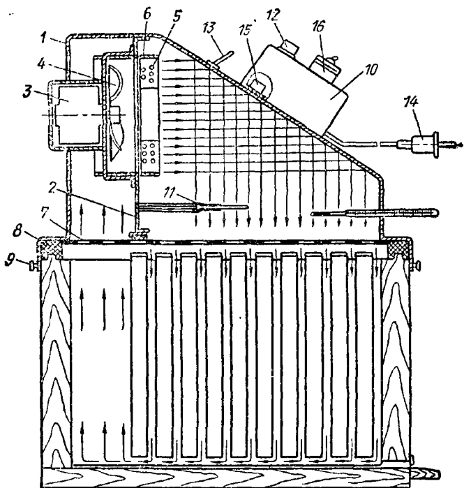
Рис. 46. Схема устройства УТП-1 в комплекте с обрабатываемым ульем
