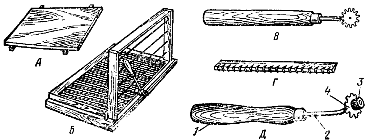
Рис. 19. Приспособления для наващивания рамок:
