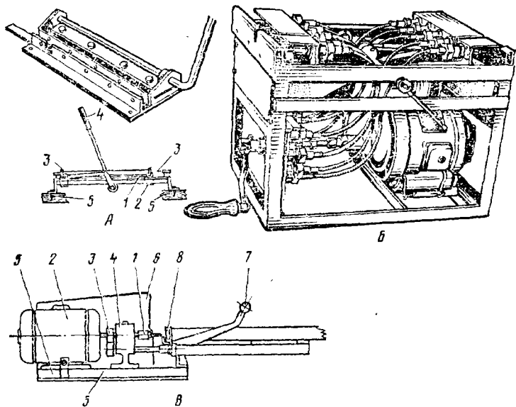
Рис. 17. Станки для сверления и прокалывания отверстий в планках рамок:
