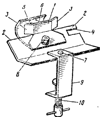
Рис. 41. Рамкоочиститель РПВ
