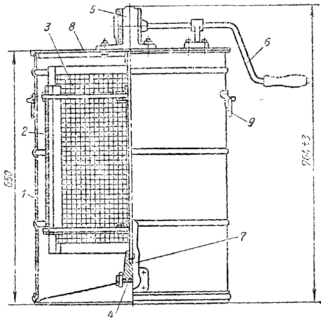
Рис. 31. Схема устройства медогонки трехрамочной хордиальной МЗРС
