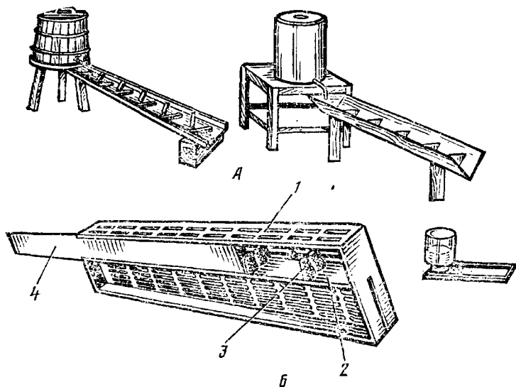
Рис. 26. Инвентарь общего назначения.
