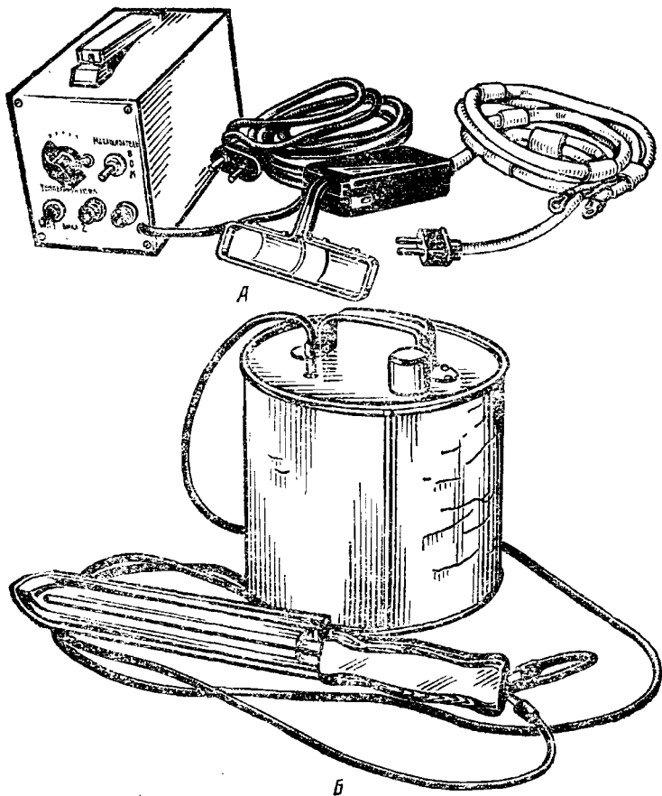
Рис. 28. Приборы для распечатывания медовых сотов:
