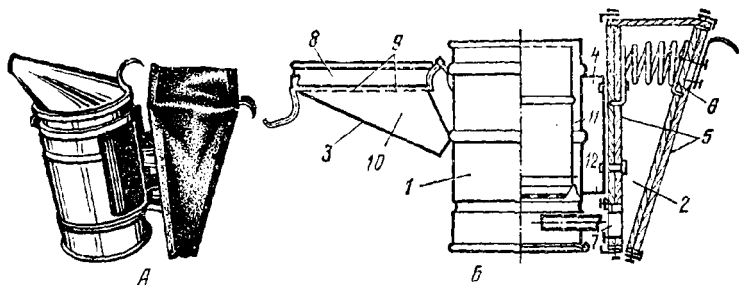
Рис. 8. Дымарь ДП: А — общий вид; Б — в разрезе
