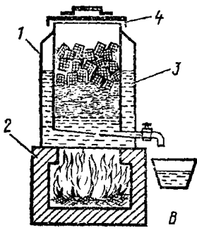
Рис. 35. Воскотопки: паровые: А — ВТП; Б — ВТ-П; В — водяная
