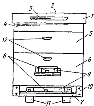
Рис. 1. Устройство улья:
