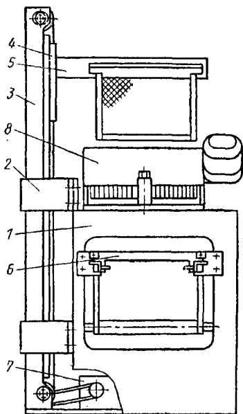
Рис. 51. Схема устройства станка для распечатывания сот М-399:
