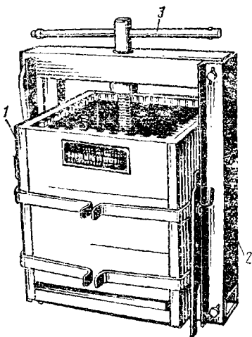
Рис. 37. Воскопресс ПВ
