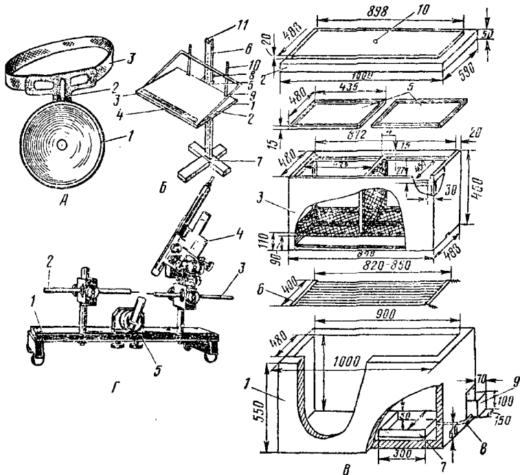
Рис. 25. Оборудование для прививки маточных личинок и осеменения пчелиных маток:
