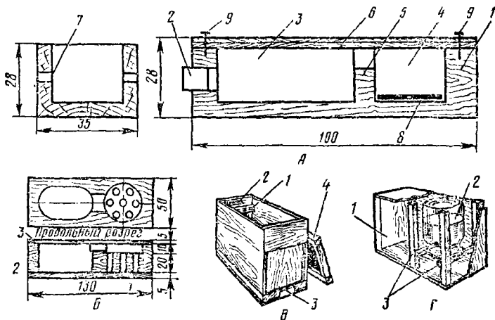
Рис. 23. Клеточки и пакеты для пересылки маток и пчел (размеры, мм):
