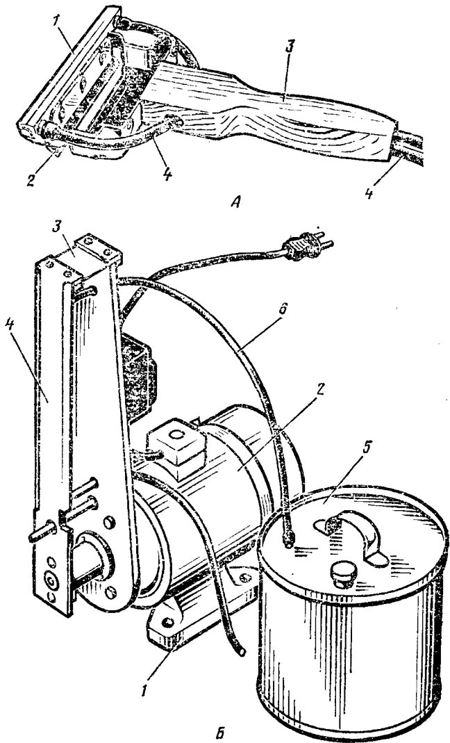
Рис. 29. Приборы для распечатывания медовых сотов: А — рубанок; Б — вибронож ВНС
