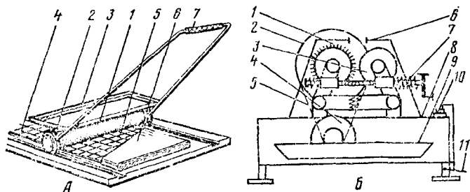
Рис. 40. Механизмы, используемые при производстве товарного прополиса:
