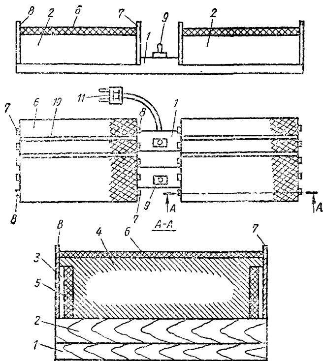
Рис. 21. Устройство для электронаващивания рамок Н. А. Пасечниченко
