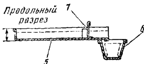
Рис. 34. Простейшие приспособления для переработки воско сырья:
