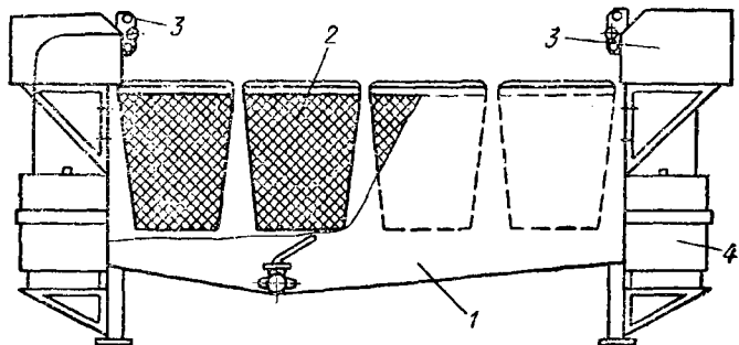
Рис. 30. Стол для распечатывания медовых сотов СПУМ
