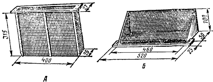
Рис. 47. Вентиляционные вкладыши и веранды:
