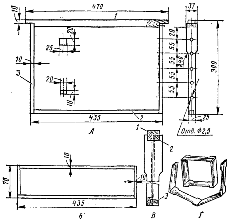
Рис. 2. Ульевые рамки (размеры, мм):
