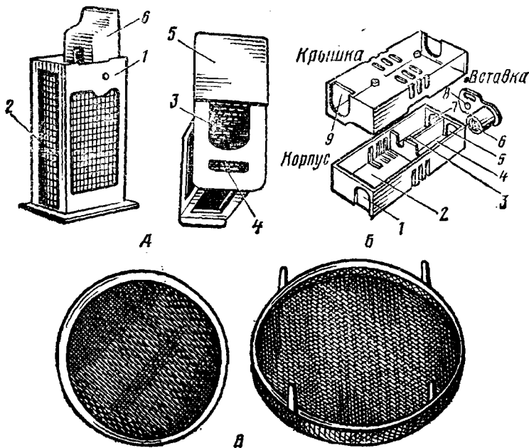
Рис. 10. Клеточки маточные:
