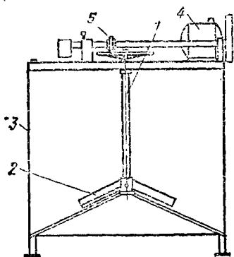
Рис. 49. Приспособление для приготовления сиропа к медогонке МР-50А
