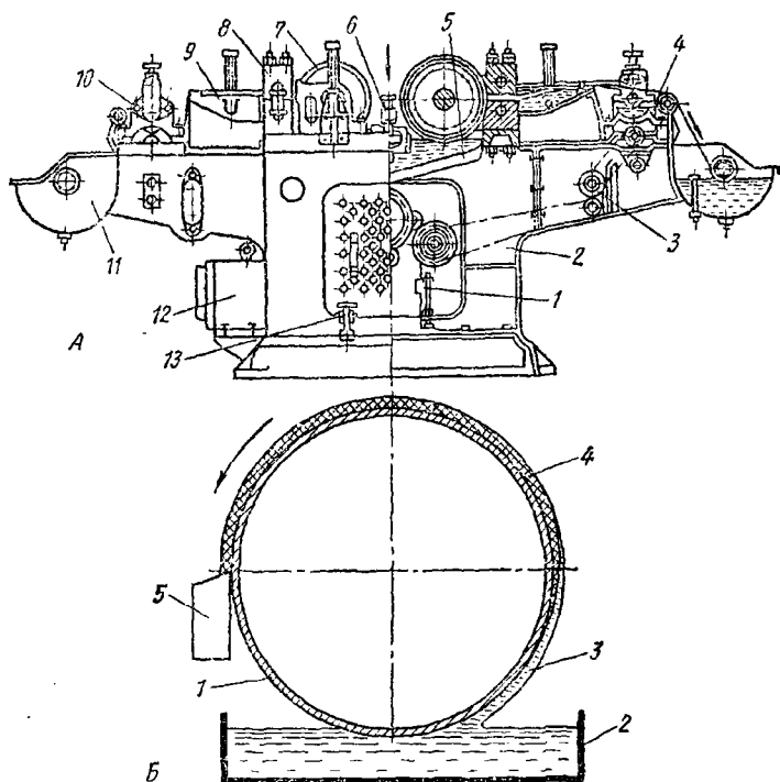
Рис. 39. Агрегат для изготовления вошины АИВ-100:
