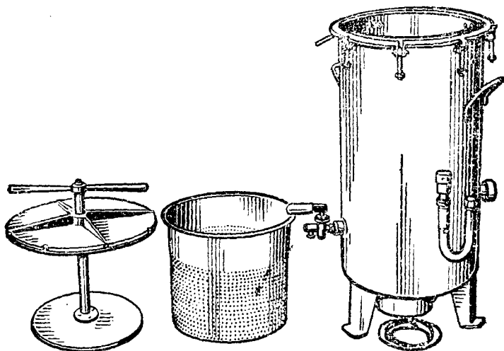
Рис. 36. Воскотопка-воскопресс ВВ-3
