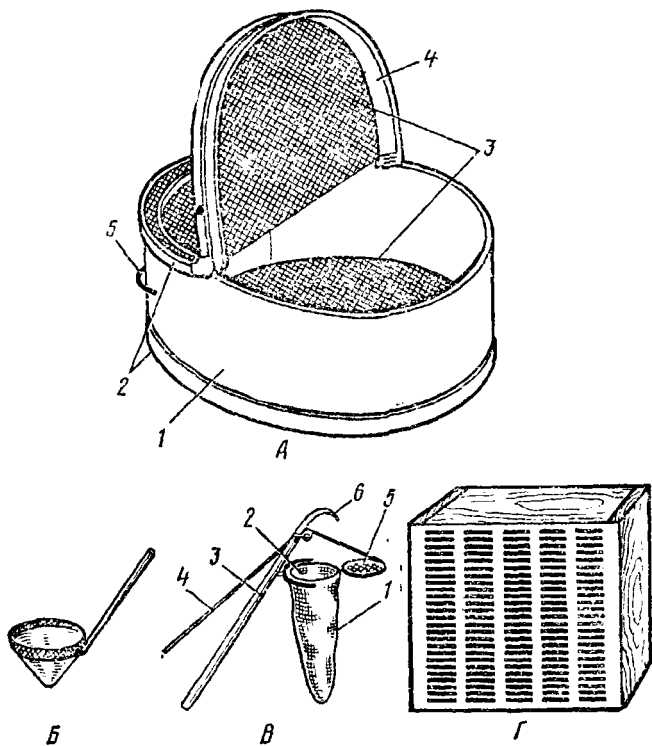
Рис. 22. Инвентарь, используемый при роении пчел:
