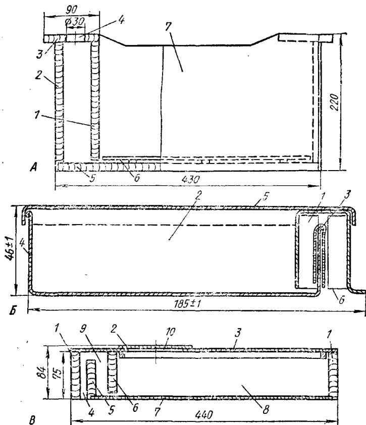
Рис. 15. Кормушки (в разрезе), размеры, мм:
