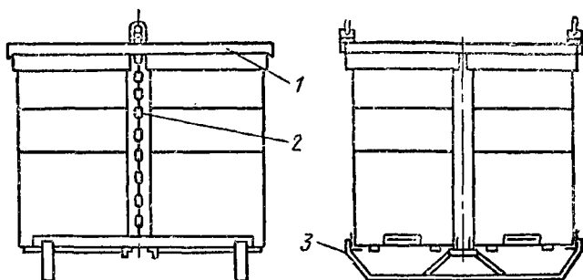
Рис. 52. Контейнер для транспортировки ульев:
