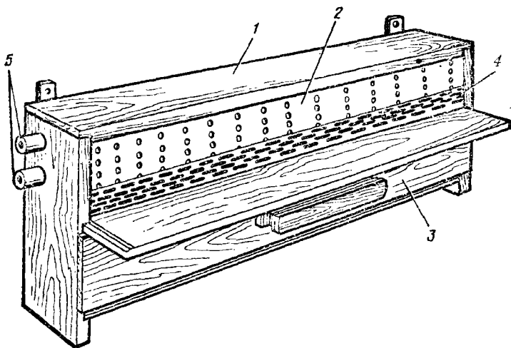
Рис. 43. Пыльцеуловитель ПУ-6
