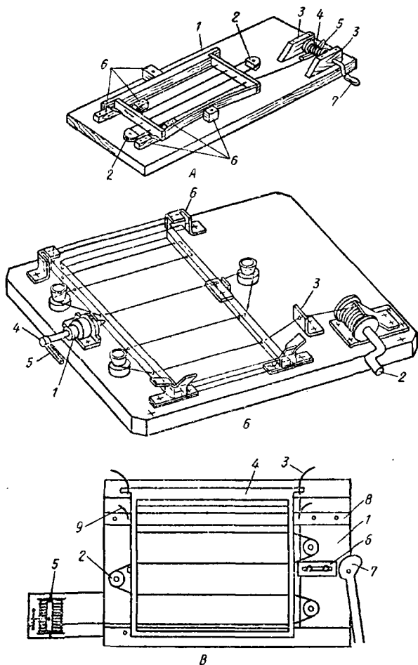
Рис. 18. Станки для натягивания проволоки на рамки:
