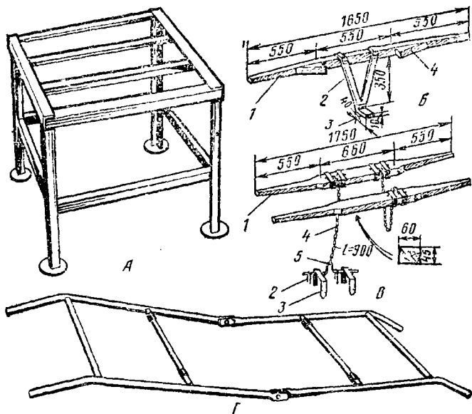
Рис. 27. Инвентарь общего назначения:
