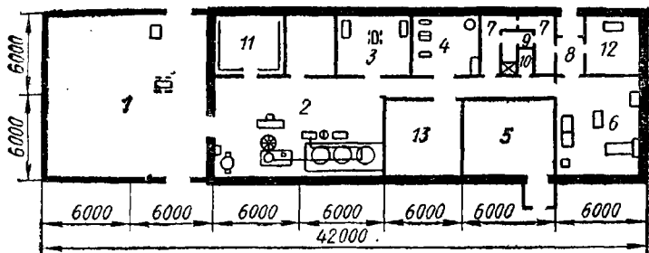
Рис. 55. План производственного корпуса на 1200 пчелиных семей (размеры, мм)
