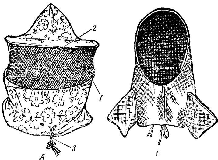
Рис. 7. Лицевая сетка:
