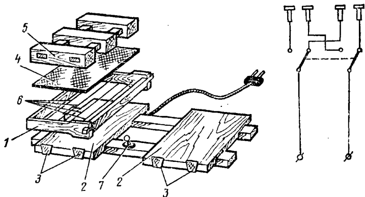
Рис. 20. Двойное лекало и схема его работы
