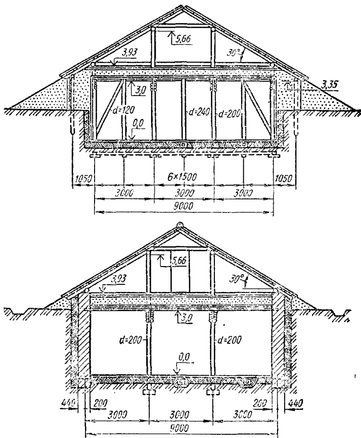
Рис. 57. Схема устройства зимовника на 250 пчелиных семей (размеры, мм):
