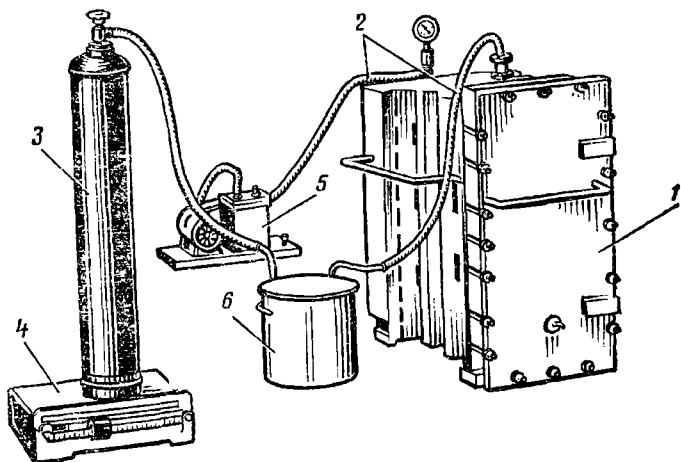
Рис. 48. Установка для дезинфекции сотов и инвентаря
