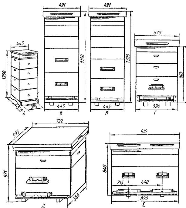
Рис. 5. Ульи:
