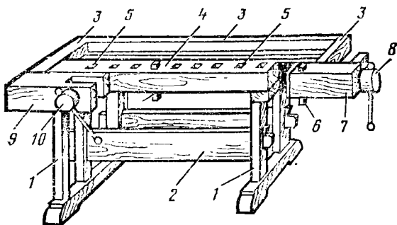
Рис. 58. Столярный верстак
