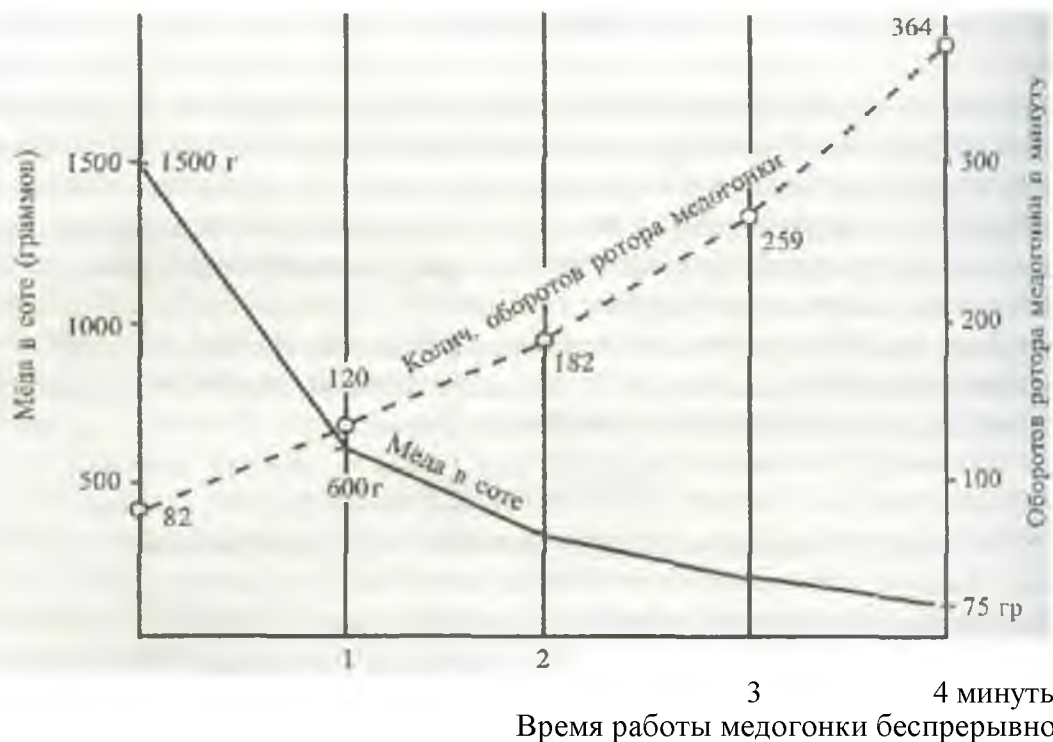
Рис.1. Диаграмма процесса работы радиальной медогонки
